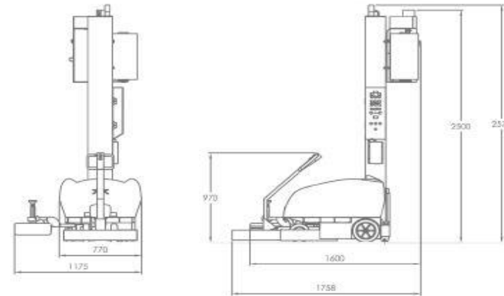
Maschinendimensionen
